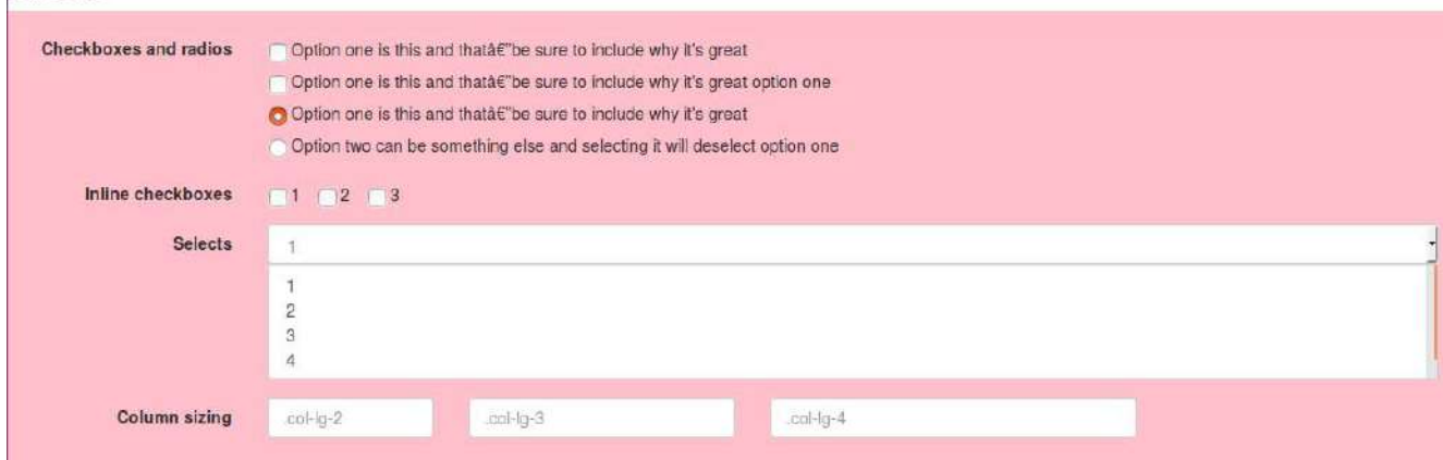
Fig. 3.13: Buttons
